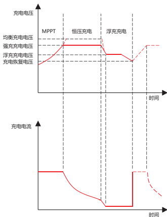
图2-2 铅酸电池充电曲线
