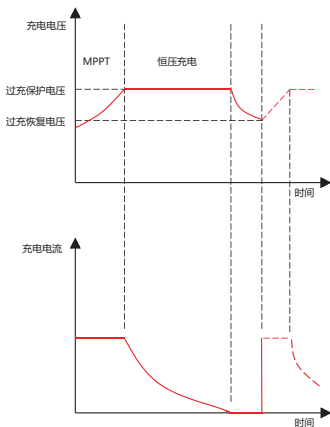
图2-3 锂电池充电曲线
