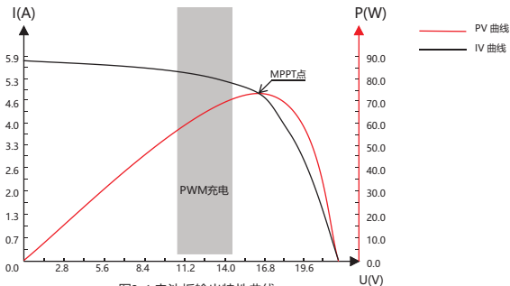
图2-1 电池板输出特性曲线
